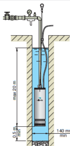
Pompe suspendue
