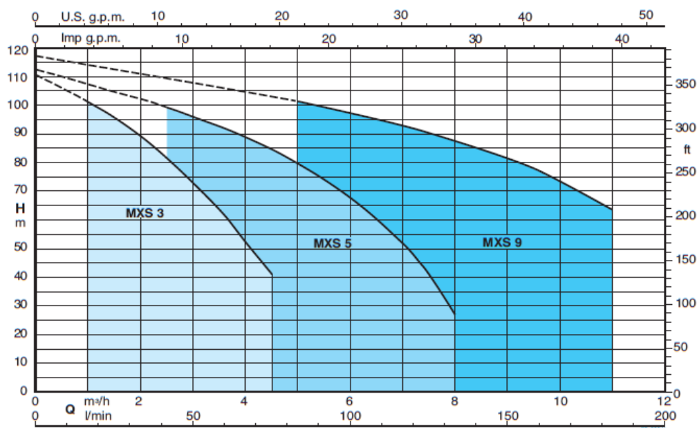
Graphique d'utilisation n \approx 2900 1/min
